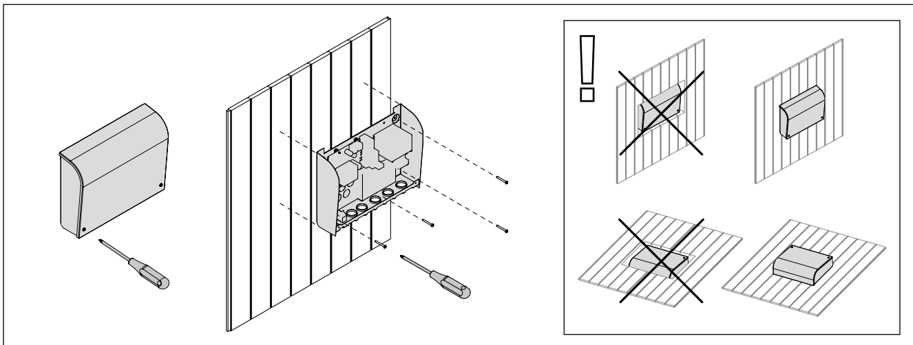
Figure 6. Opening the power unit cover and mounting the unit Abbildung 6. Öffnen der Abdeckung der Leistungseinheit und Wand-/Deckenmontage des Geräts
